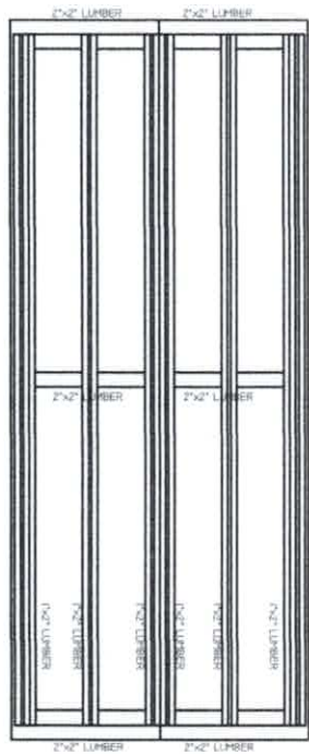
FRAMING PLAN SCALE 1:10 MET
