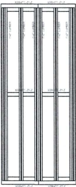
FRAMING PLAN SCALE: 1/8" = 1'-0"
